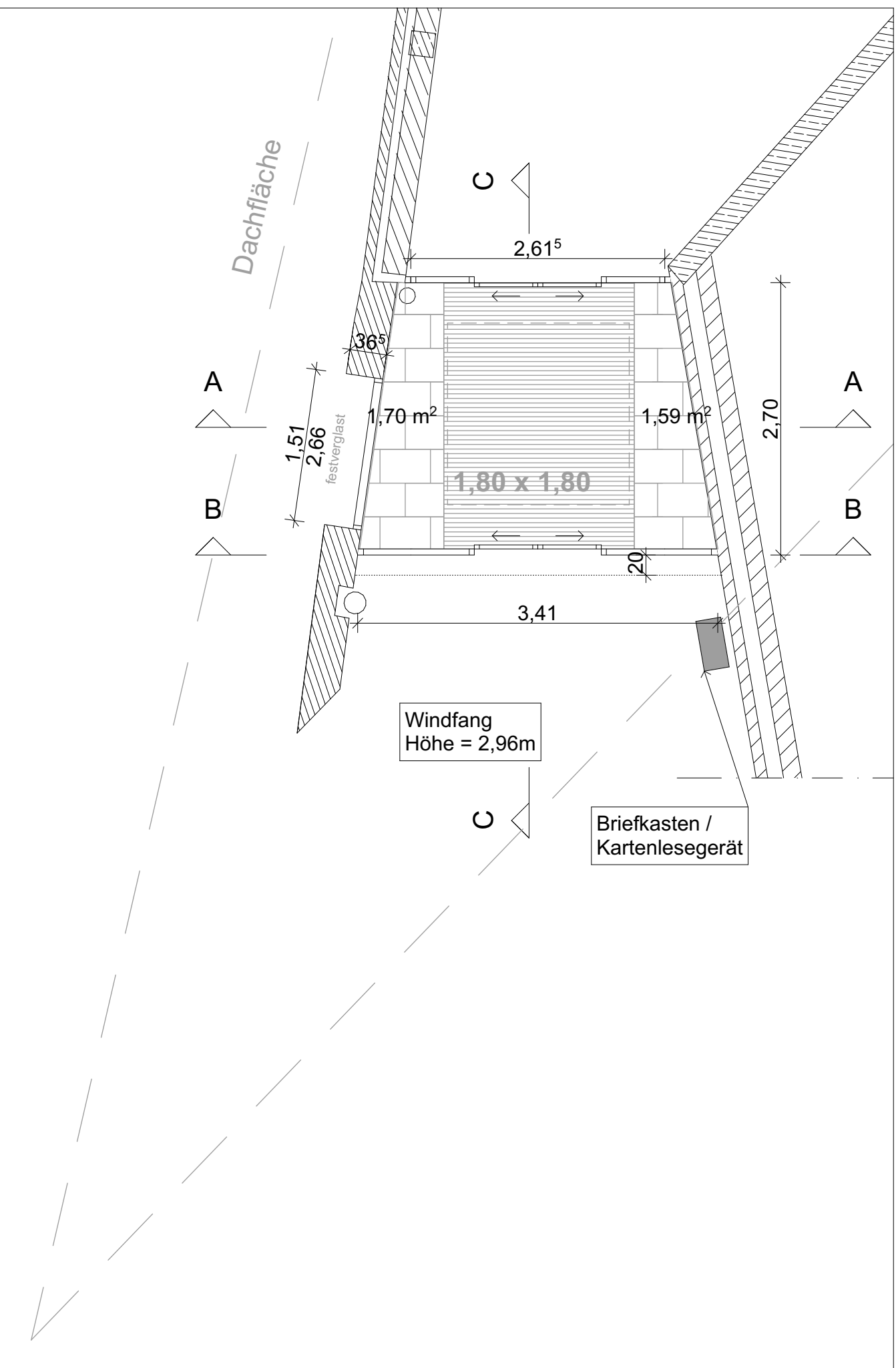
Auszug Windfang M 1:50
