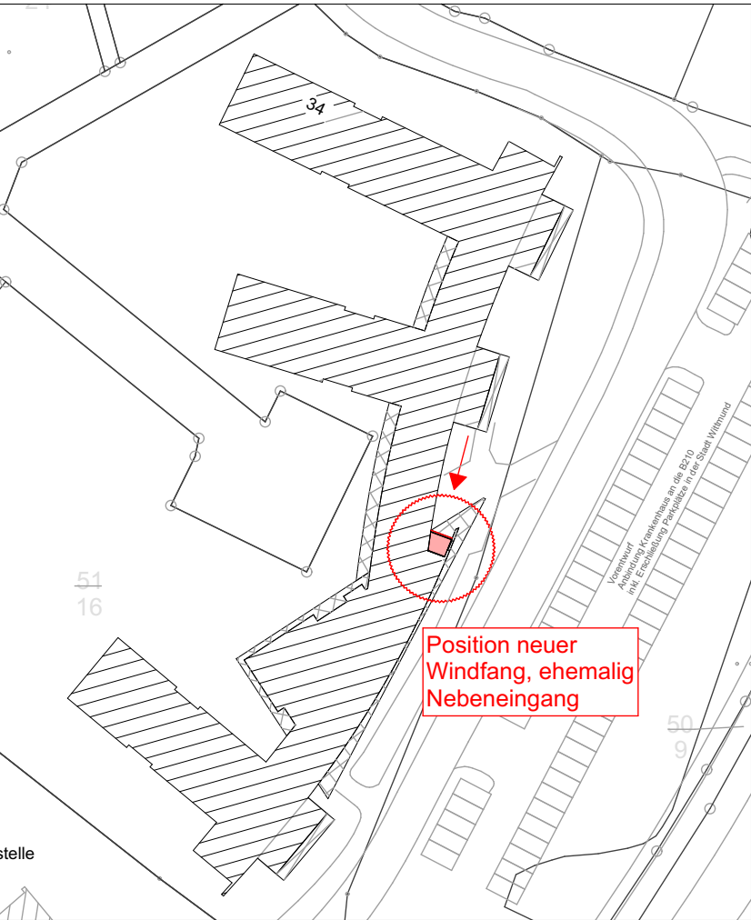
Auszug Lageplan Liegenschaftskataster M 1:1000
